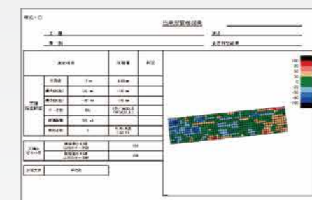
出来形管理図
